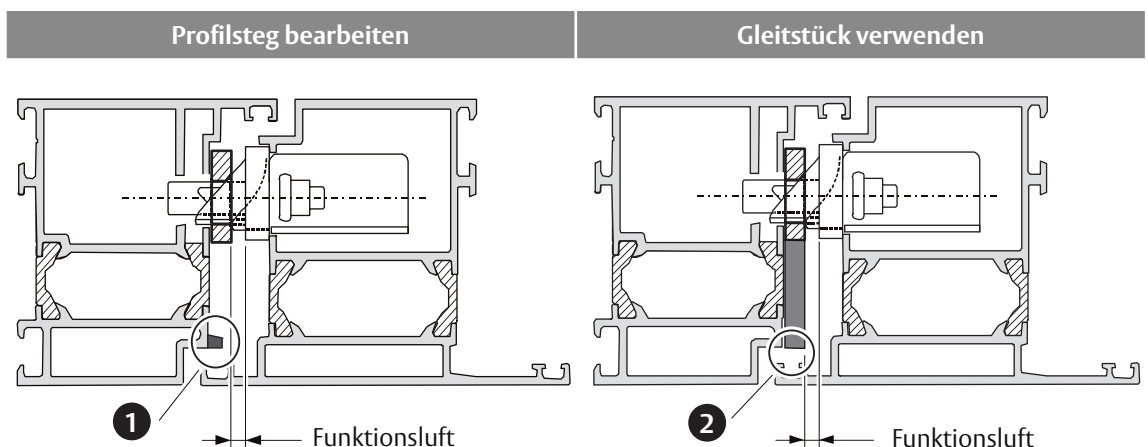
Abb. 19: Profilsteg nachbearbeiten und Gleitstück verwenden
