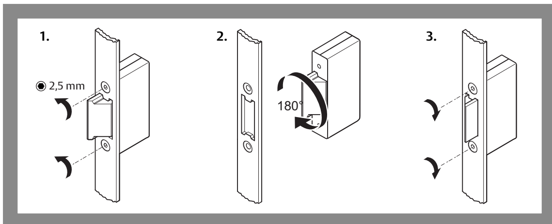
Fig. 10: Adattamento della direzione di chiusura della serratura a scrocco 807-10 al saliscendi
