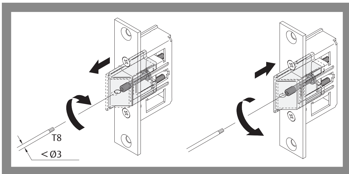
Fig. 11: Regolazione della corsa scrocco della serratura a scrocco 807-10
