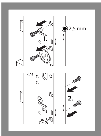
Afb. 12: Paniekzijde instellen
