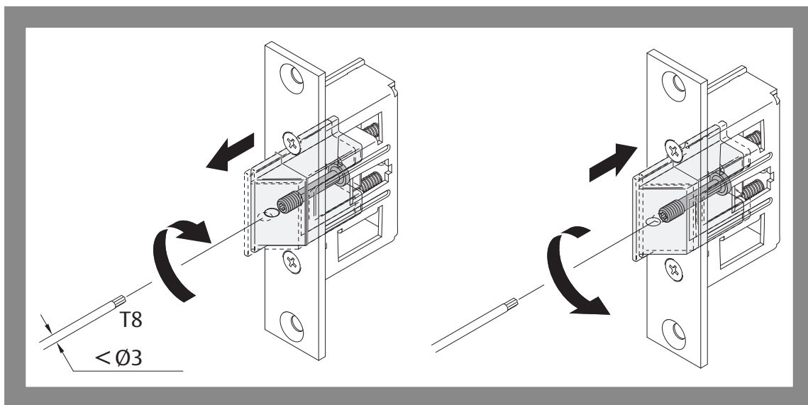
Fig. 11 : Régler la course du pêne sur la serrure à pêne demi-tour 807-10
