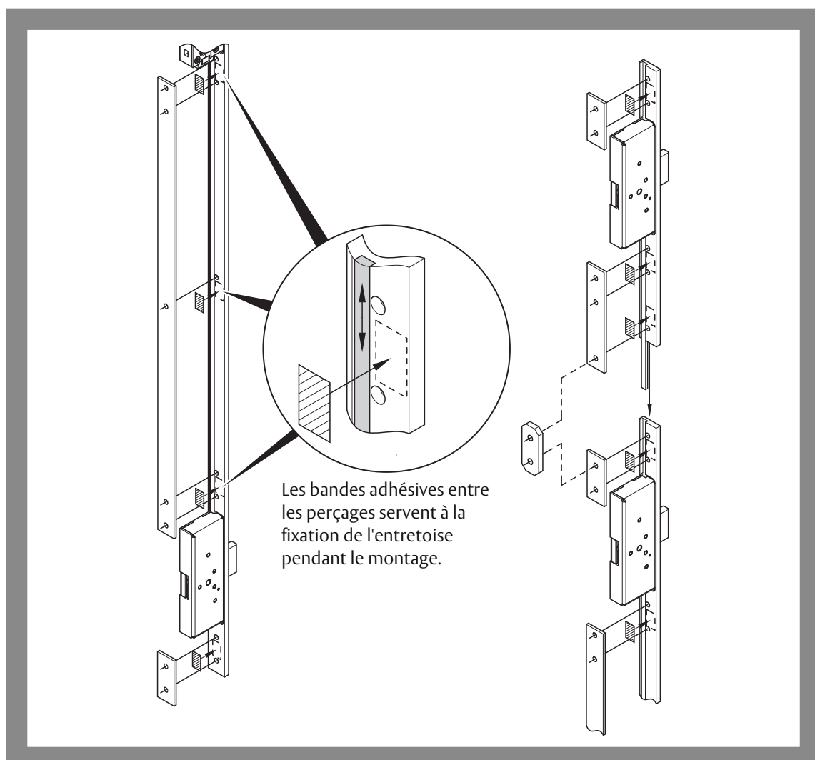
Fig. 22 : Utilisation d'entretoises
