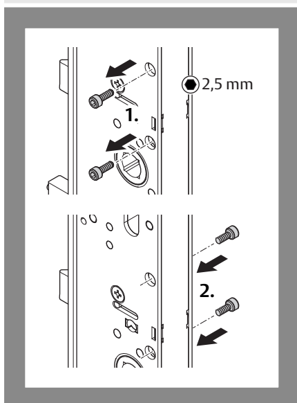
Fig. 12 : Régler le côté anti-panique
