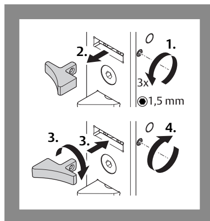
Abb. 9: Steuerfalle drehen
