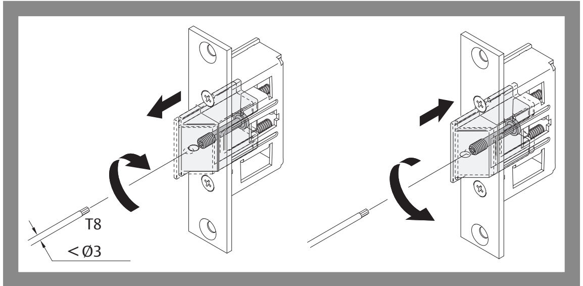
Abb. 11: Fallenausschluss des Fallenschloss 807-10 einstellen
