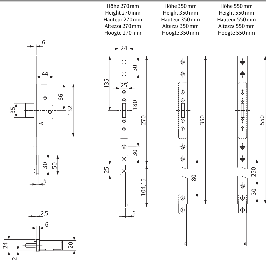
Abb. 27: Abmessungen Zusatzriegel
