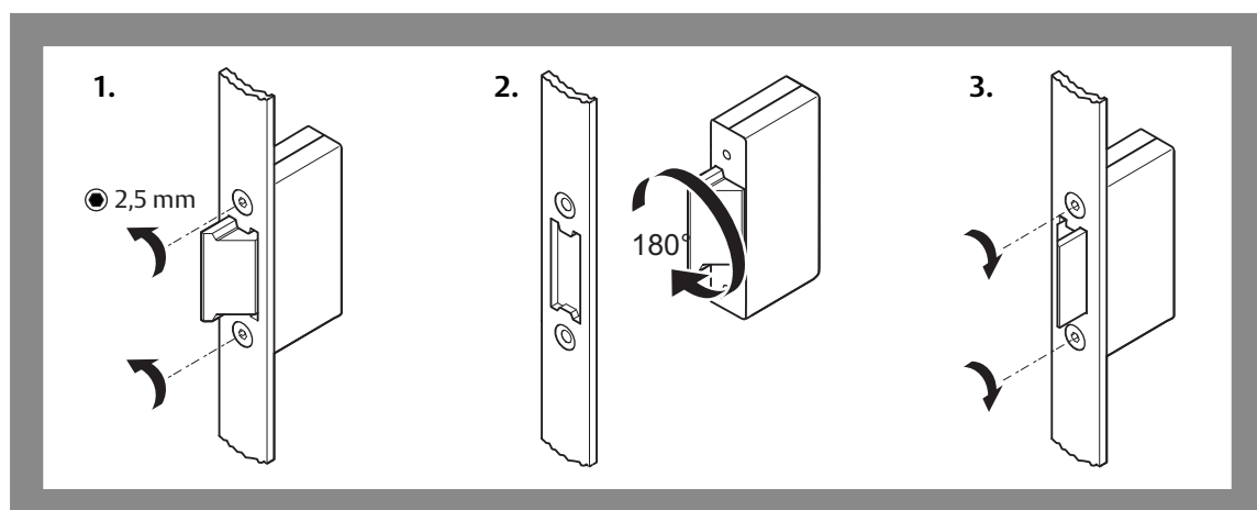
Fig. 10 : Adaptation du sens d'ouverture de la serrure à pêne demi-tour 807-10 au pêne pilote
