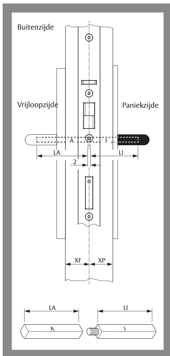
Afb. 14: en deurkruk
