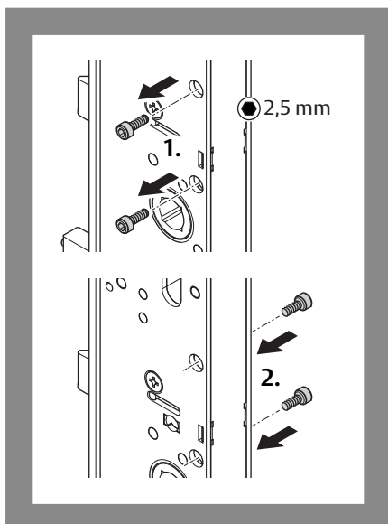
Abb. 12: Panikseite einstellen
