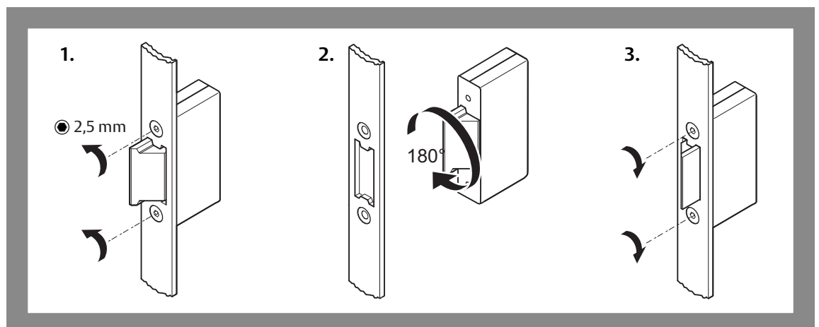
Abb. 10: Anschlagrichtung des Fallenschloss 807-10 an Steuerfalle anpassen
