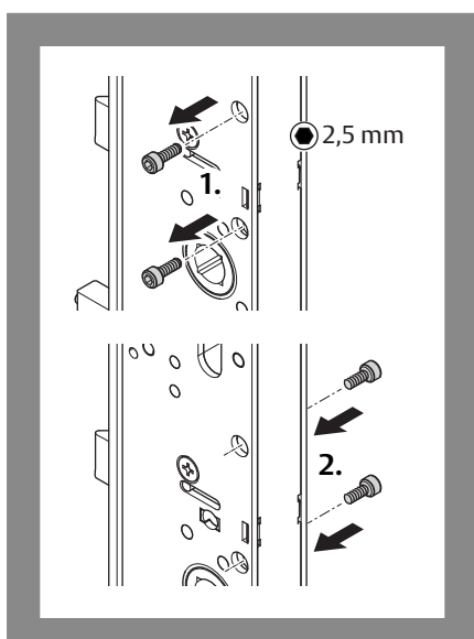
Fig. 12: Regolazione del lato antipanico
