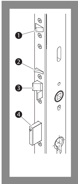
Abb. 4: Türkontakt Steuerfalle Schlossfalle Riegel
