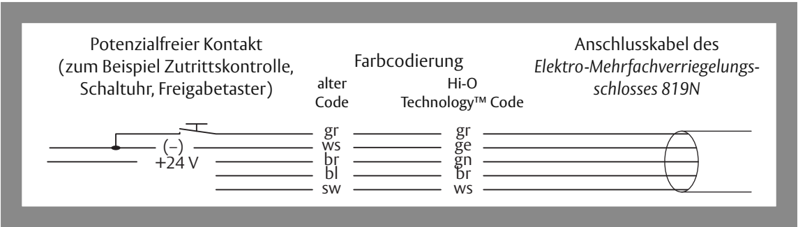
Abb. 13: Anschlussplan
