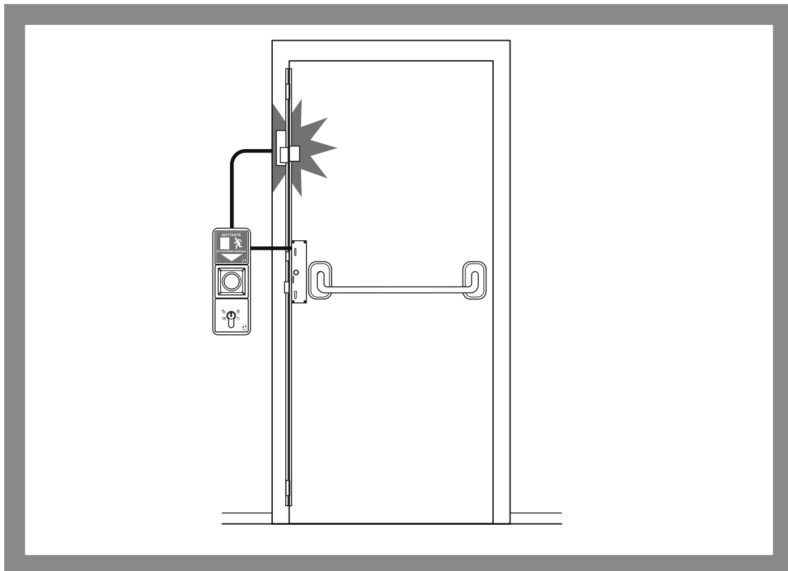
Afb. 6: Vluchtdeurbeveiliging met effectvluchtdeur- besturingsterminal 1385
